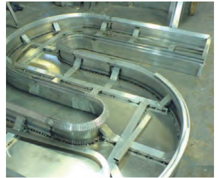
Ejemplo de rótulo de letras corpóreas realizadas con perfil de tensión
