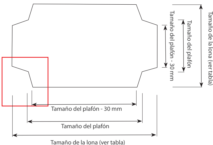
Corte del frontal flexible
